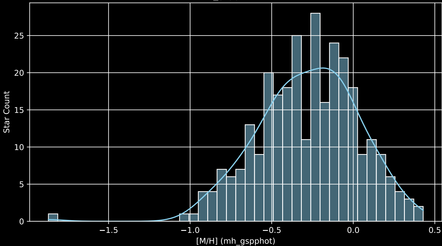
GALAH DR4 Field: [6924] [M/H] (mh_gspphot) (n= 296)
