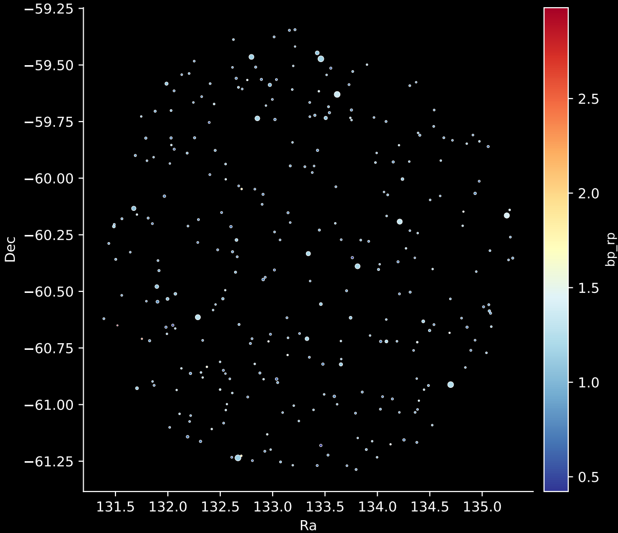
GALAH DR4 Field: [6924] Stars: 299
