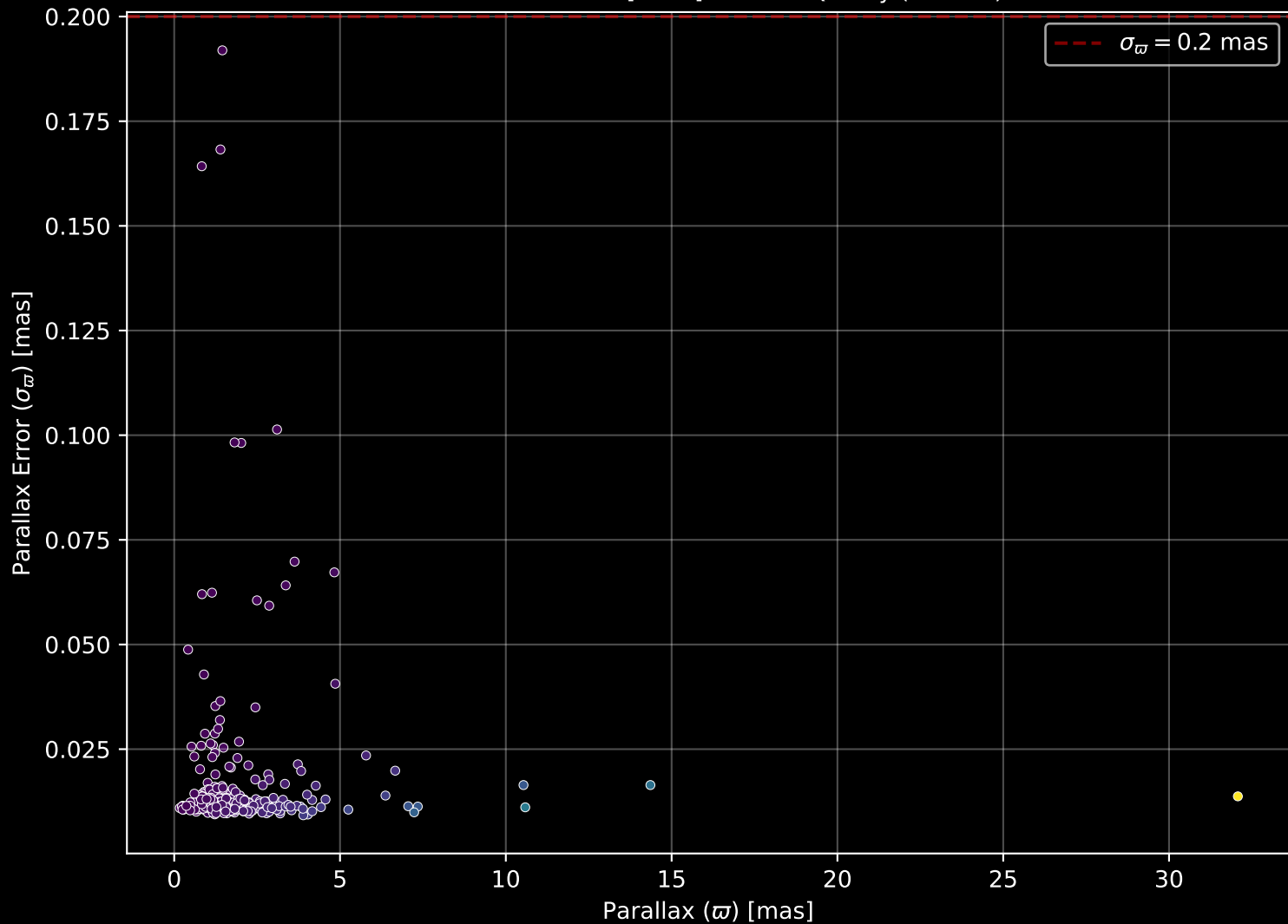
GALAH DR4 Field: [6924] Parallax Quality (n= 299)
